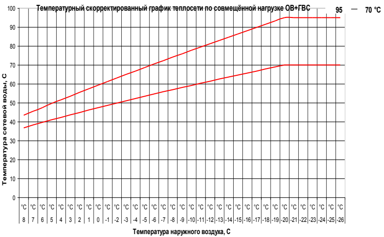
Температурный режим работы наружной теплосети 95 — 70 °С по графику центрального качественного регулирования по смешанной нагрузке отопления и ГВС
