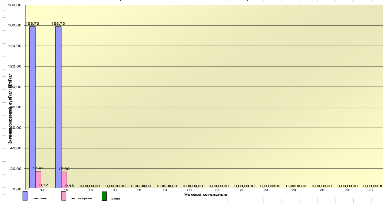
Значения удельных расходов топлива, эл. энергии и воды на выработку 1 Гкал тепловой энергии ( по котельным № 14 -- 15 )
