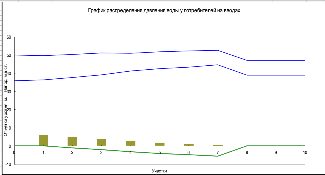
Расчетные давления воды в характерных точках теплосети :
